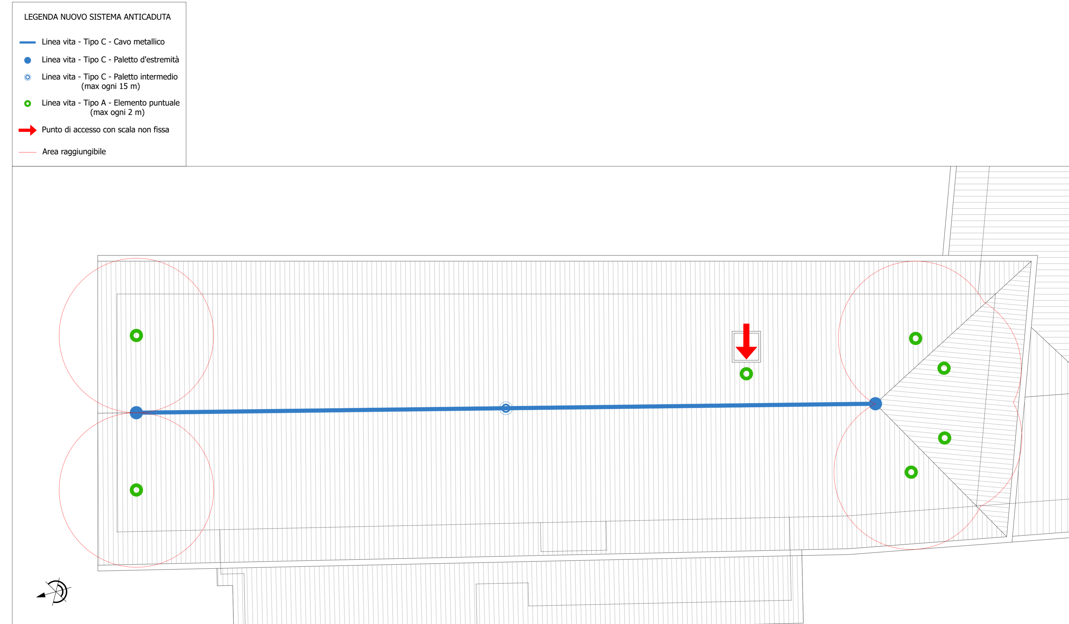
SCHEMA NUOVA LINEA VITA - FABBRICATO A Scala 1:50
