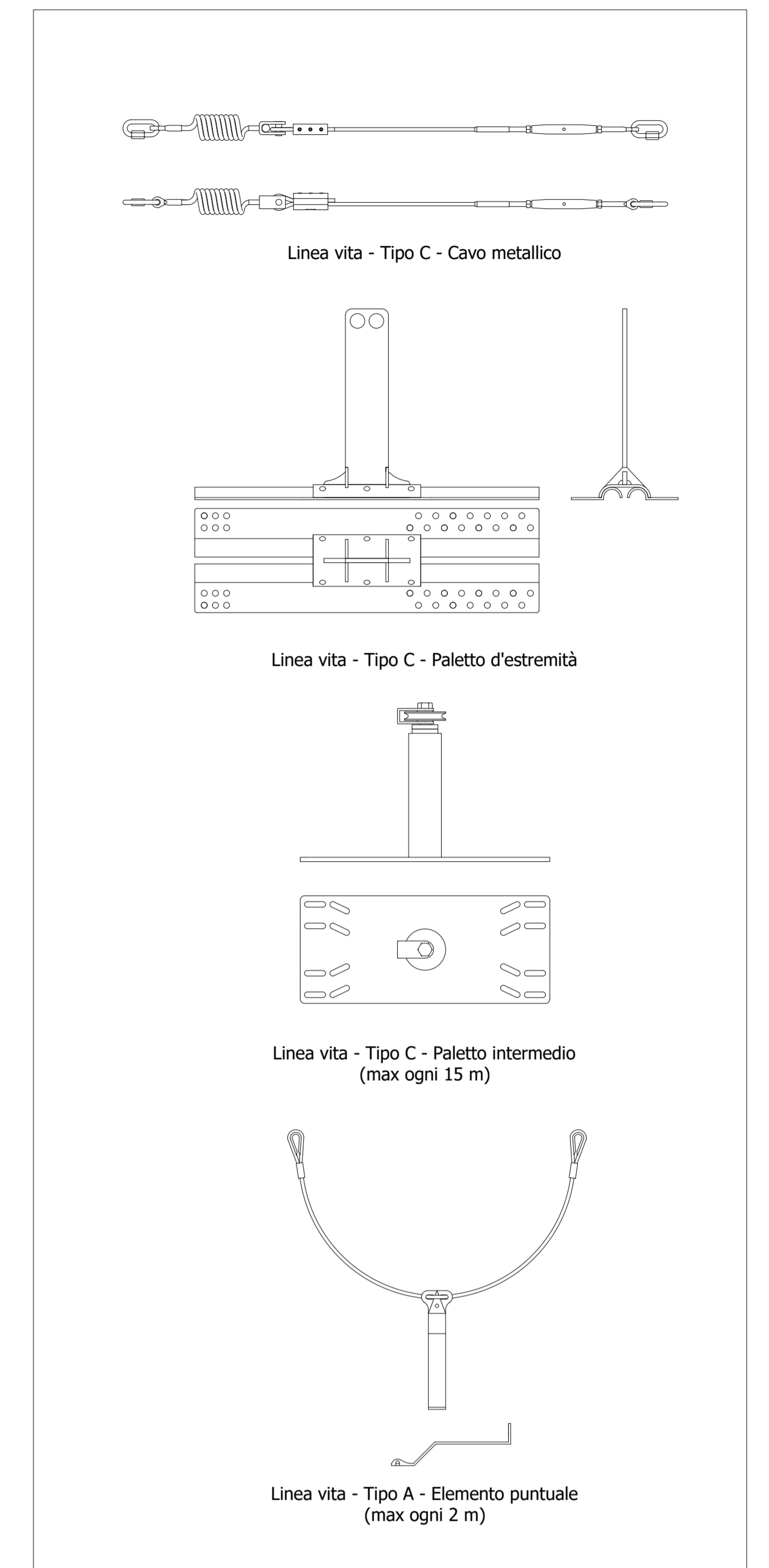
ELEMENTI LINEA VITA Scala 1:10
