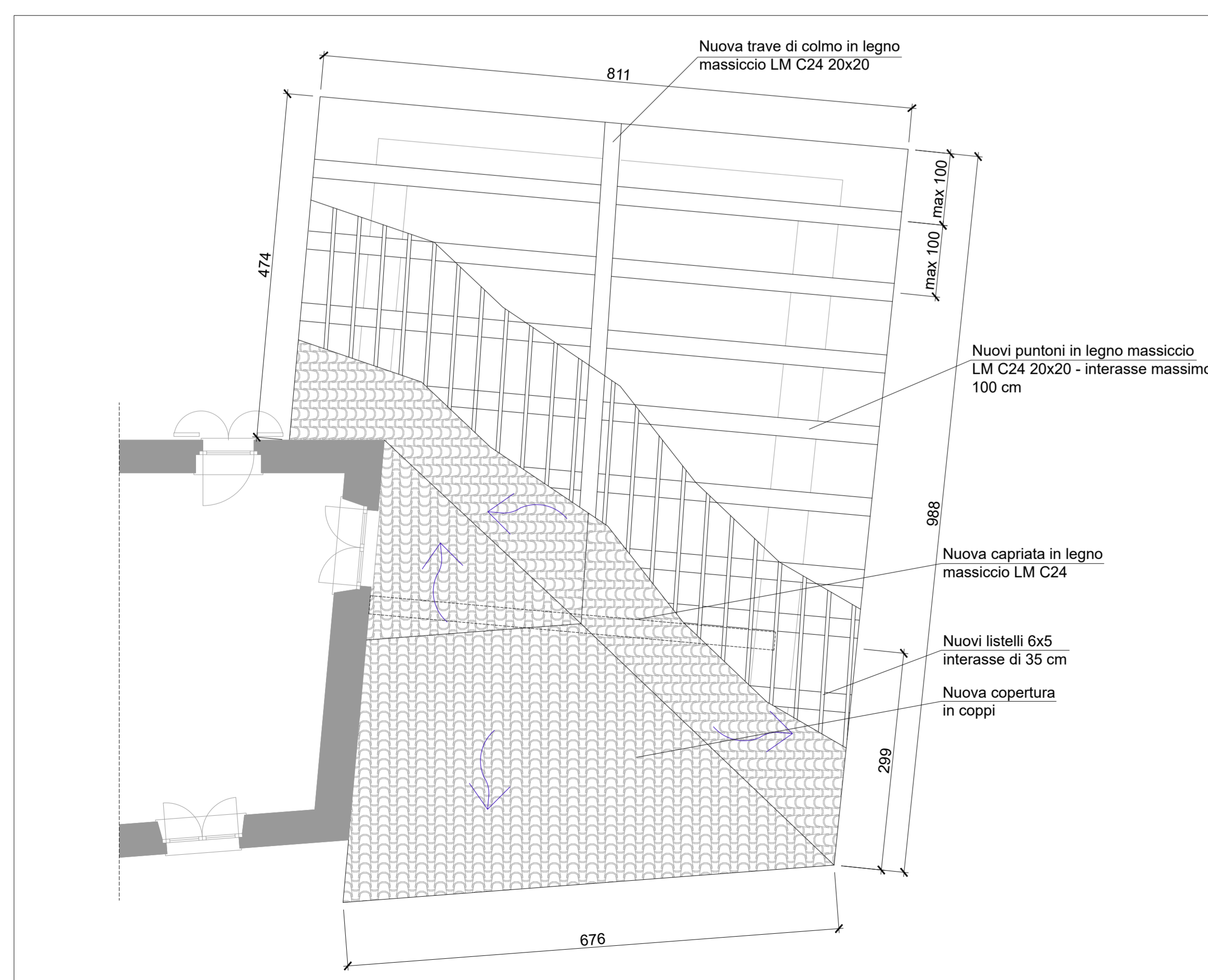
SCHEMA COPERTURA - FABBRICATO B Scala 1:50
