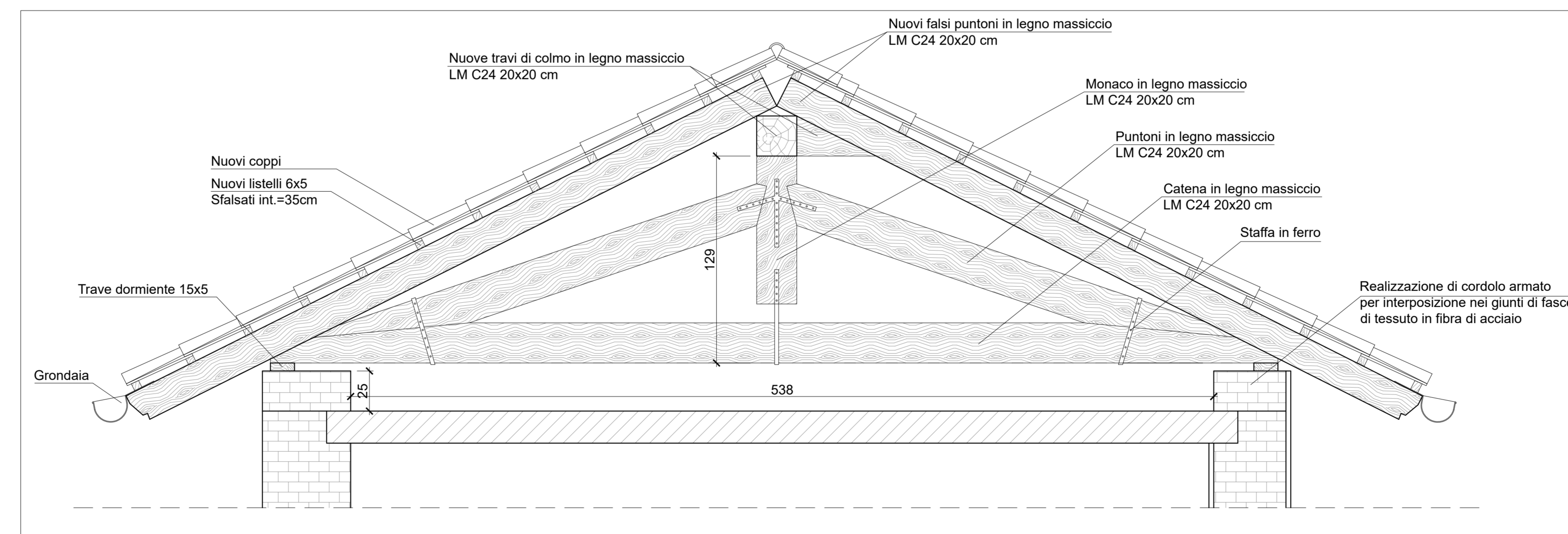
DETTAGLIO COPERTURA - FABBRICATO B Scala 1:20
