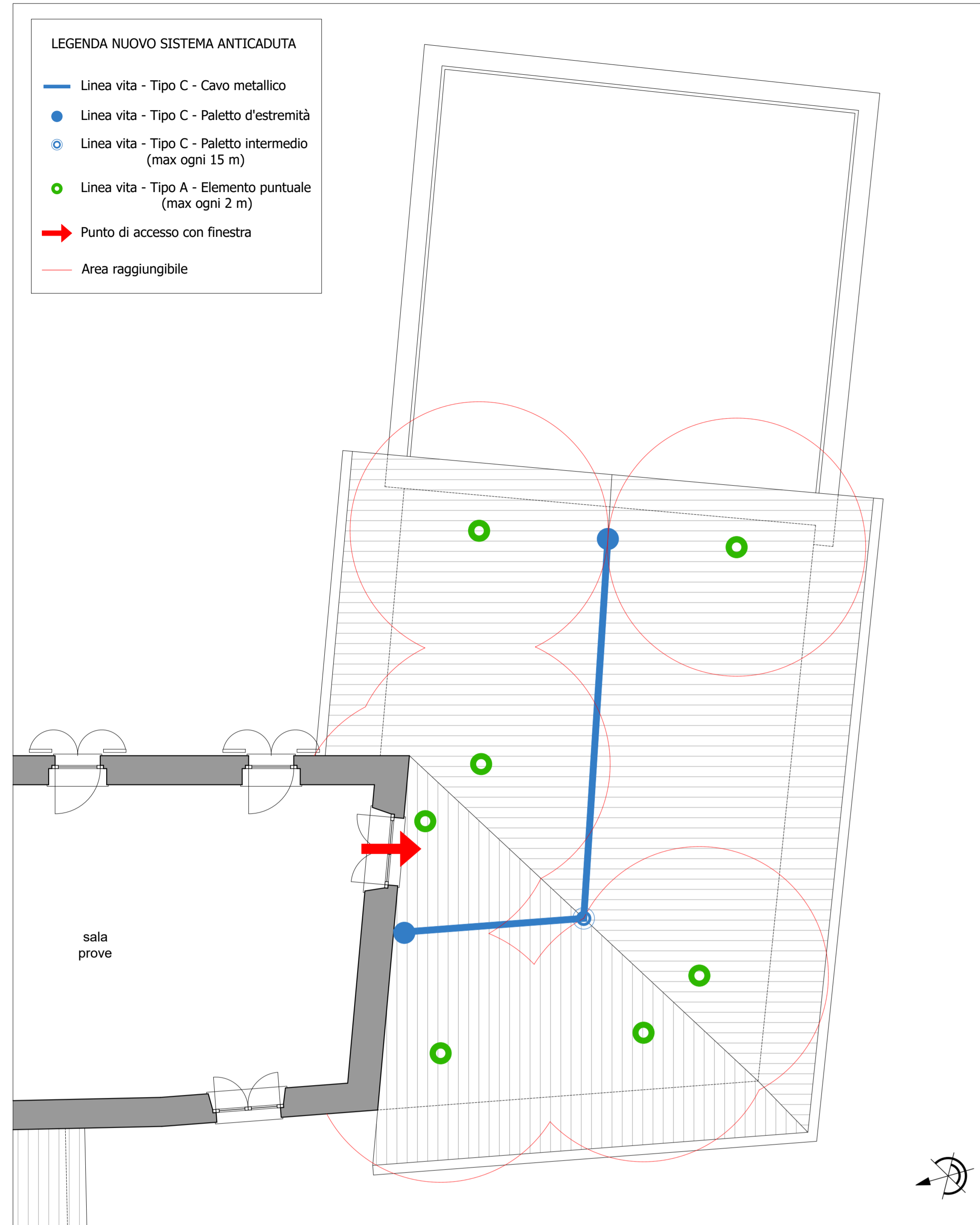
SCHEMA NUOVA LINEA VITA - FABBRICATO B Scala 1:50
